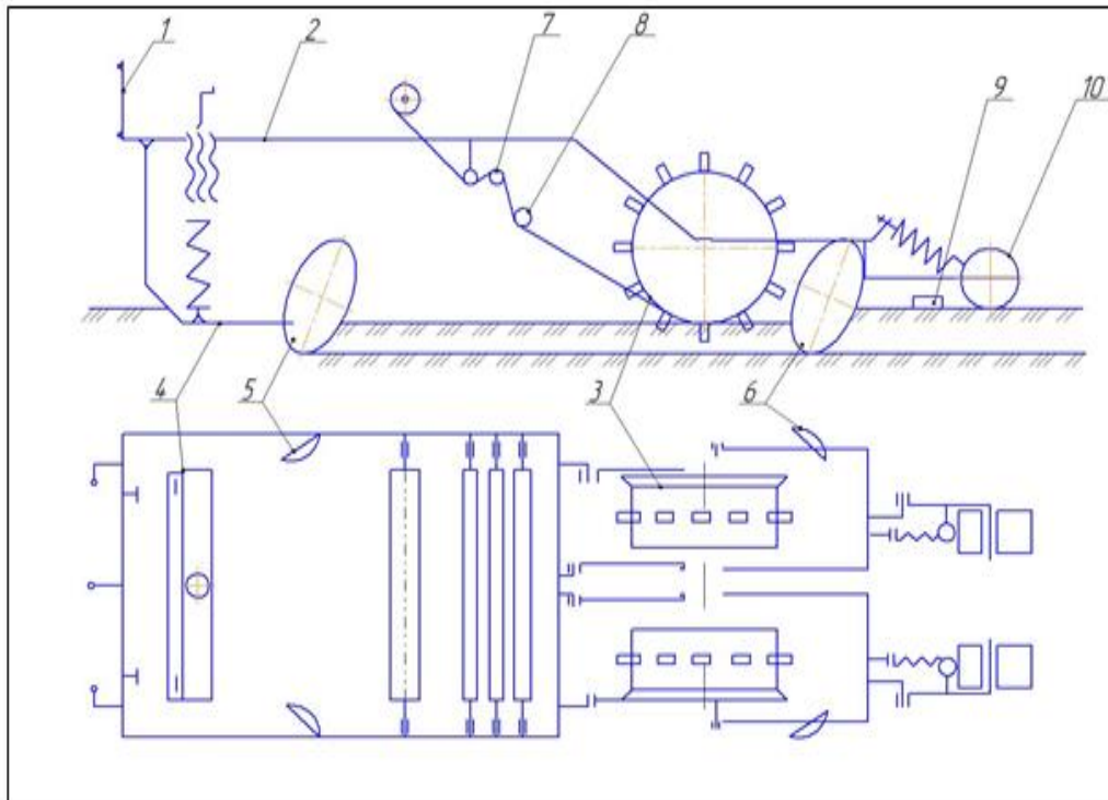
Пленка остига чигит экадиган сеялканинг технологик схемаси
